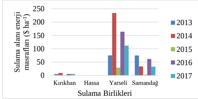
Şekil 4. Sulama alanı enerji masrafları(B5)
